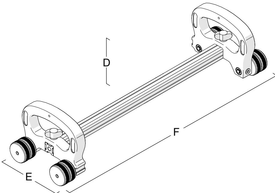
Fig. 2 - Frame dimensions
