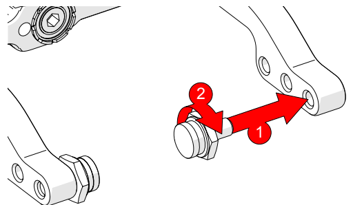
Fig. 65 - Pivot buttons
